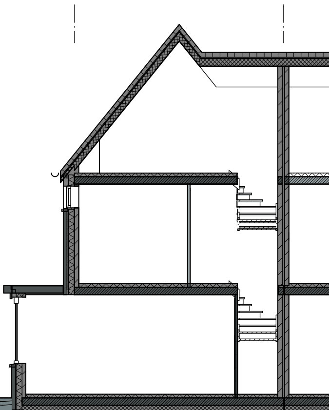
DOORSNEDE
