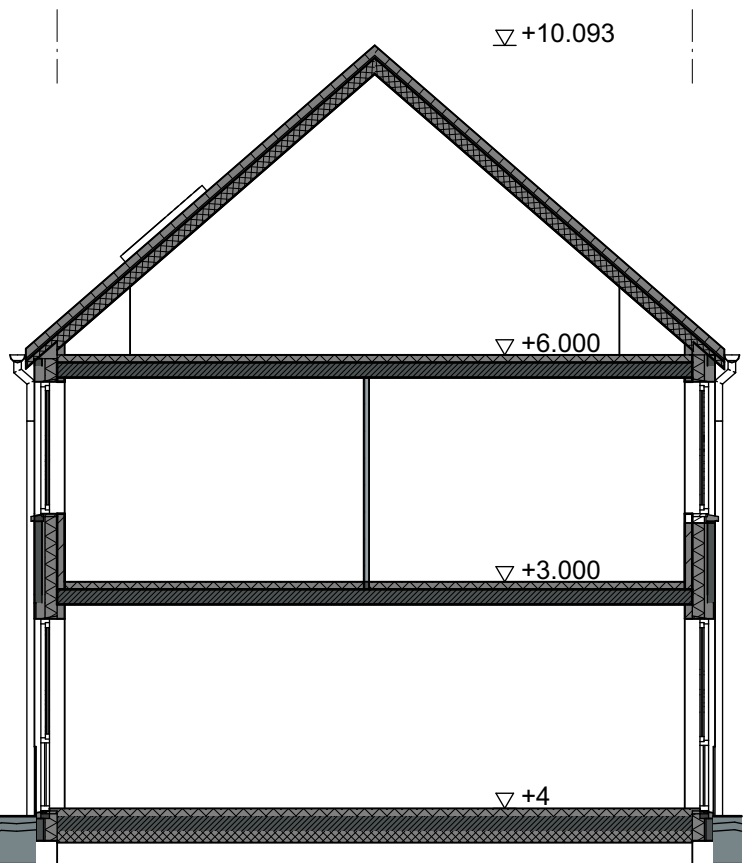
DOORSNEDE
