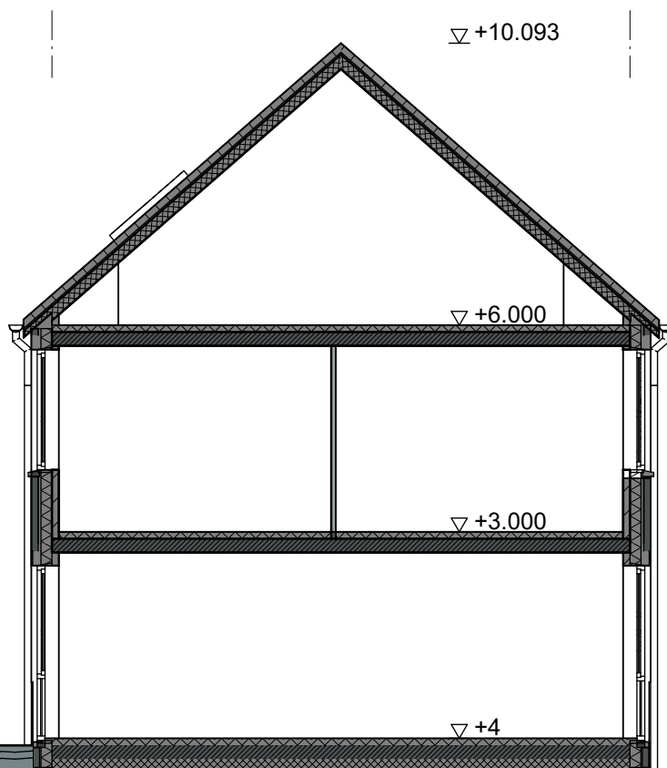
DOORSNEDE
