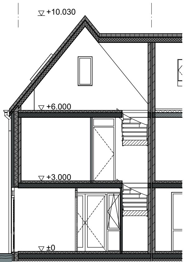
DOORSNEDE
